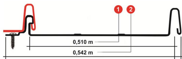
1 - Gesamtbreite 2 - Nutzbreite
